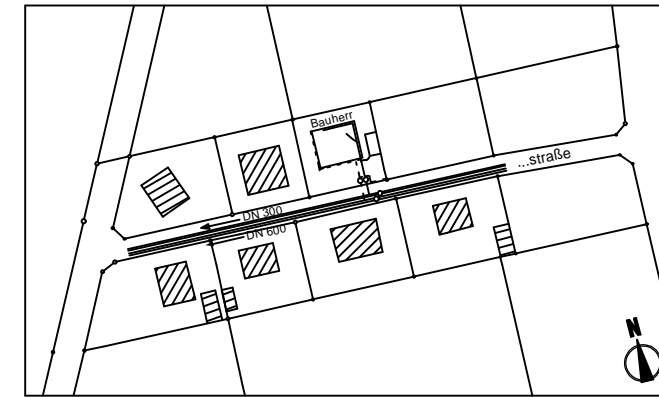
Lageplan M 1:1000
